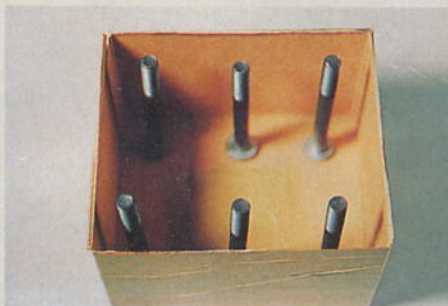
Das Gehäuse ist eine Pappschachtel; zur Stabilisierung werden sechs Paßstifte mit eingegossen.
