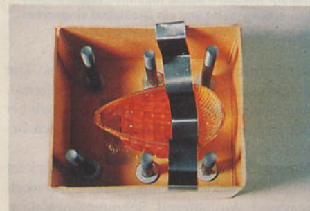
Das Glas muß (für den zweiten Abguß!) waagrecht und tief genug in der Form plaziert werden.
